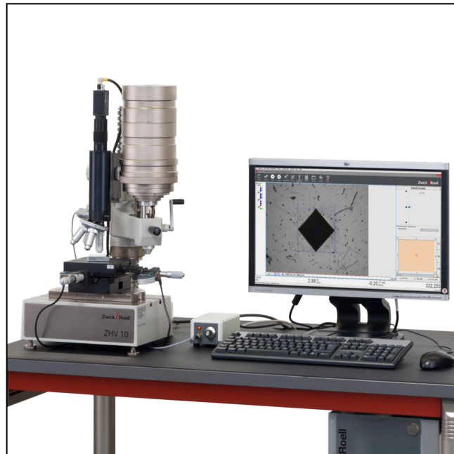
Zukunftssicher, aber mit altbewährter Bedienung: ZwickRoell ZHV10 mit testXpert hardness edition
